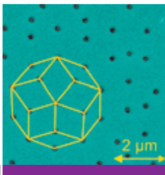
Rasterelektronenmikroskopische Aufnahme eines Nb Dünnsfilms mit nanostrukturierten Löchern (Antidots). Die Antidots sind auf den Kreuzungspunkten eines 5-faltigen Penrose-Gitters (gelbe Linien) platziert.
