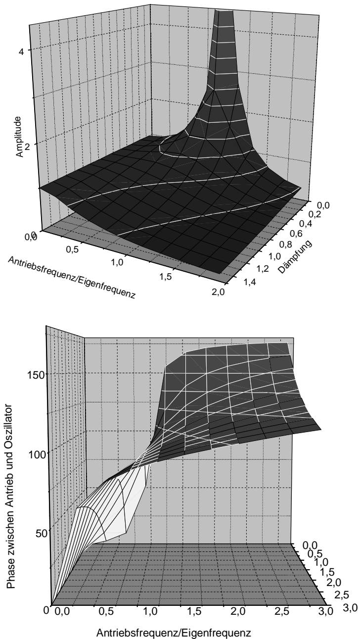
Abbildung 5 Amplitude und Phase bei erzwungenen Schwingungen in Abhängigkeit vom Verhältnis von Antriebsfrequenz zu Eigenfrequenz des freien Schwingers und der Dämpfung.
