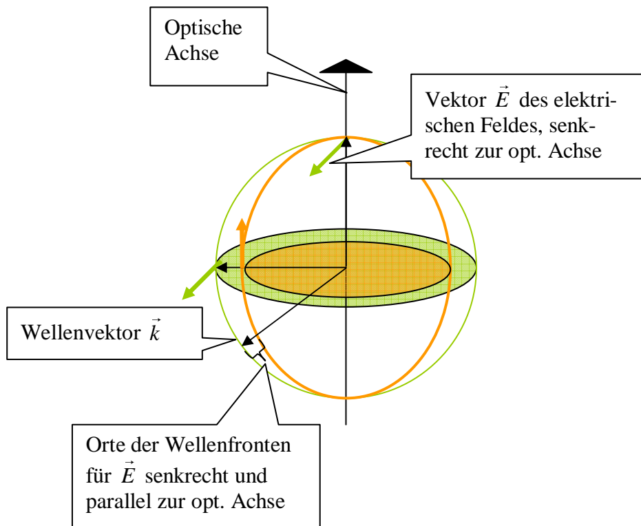
Abbildung 6 Ausbreitungsgeschwindigkeiten in Abhängigkeit von der Einfallsrichtung für den außerordentlichen Strahl (orangefarbenes Ellipsoid, „Indikatrix“) zu einem optisch anisotropen, einachsigen positiven Kristall: Der Betrag eines Vektors vom Mittelpunkt bis zur Oberfläche des Ellipsoids zeigt die Geschwindigkeit des außerordentlichen Lichts, wenn es sich in Richtung des Vektors ausbreitet. Die Ausbreitungsgeschwindigkeit des ordentlichen Lichts ist für alle Richtungen gleich (grüne Kugel). Nähert sich die Ausbreitungsrichtung des außerordentlichen Lichts der optischen Achse, dann werden die Unterschiede zwischen beiden Strahlen kleiner.
