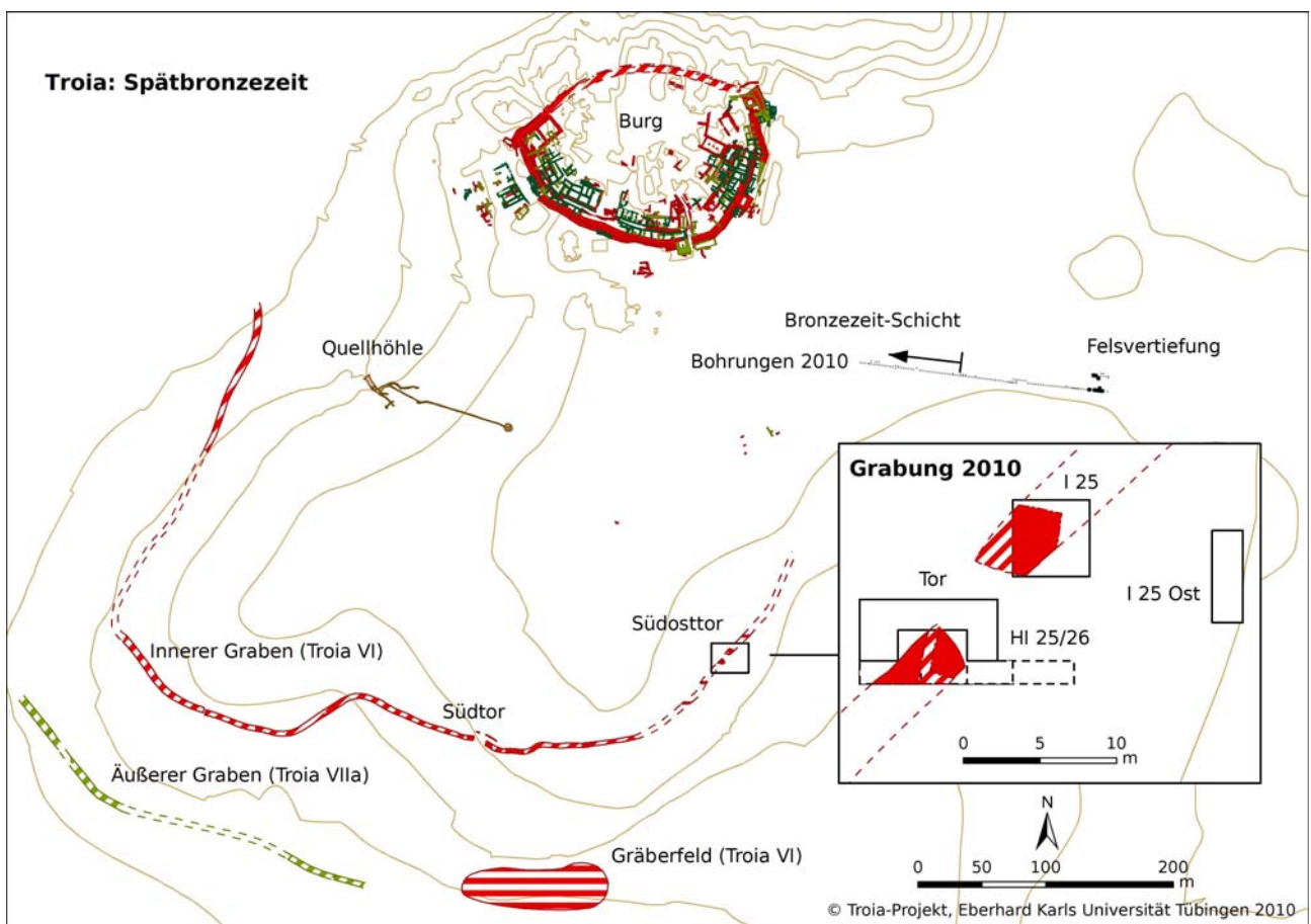
1. Plan des spätbronzezeitlichen Troia mit Grabungen und Bohrungen 2010. Quelle: Universität Tübingen.
