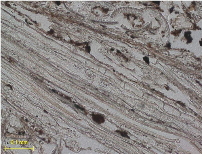
Mikrofoto eines geologischen Dünnschliffes der Pflanzenbettungen (Maßstab in der linken unteren Bildecke 0,1mm). Die laminierten Überreste der Blätter und Stengel sind hier als kieselsäure-haltige Fossilien erhalten. Diese Pflanzenbettungen datieren auf 77.000 Jahre vor heute. Foto Miller.
